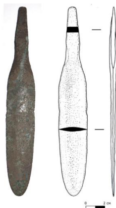
Рис. 2. Двулезвийный нож-кинжал (1). Случайная находка. Поселение бронзового века Аккаин [Fig. 2. Double-edged knife-dagger (1). A random find. The Bronze Age settlement of Akkain]
