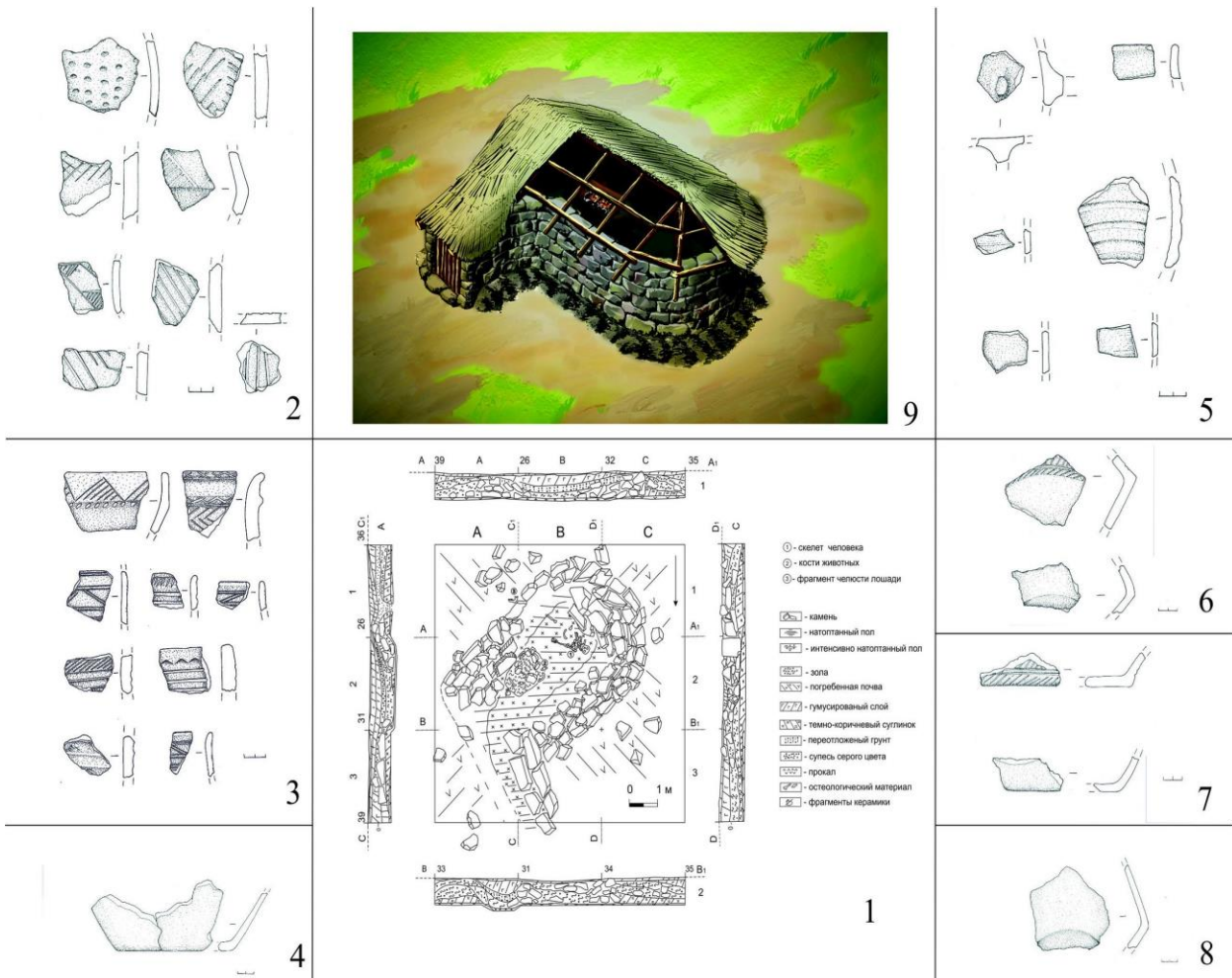
Рис. 3. Поселение Шагалалы II. Третий тип дома с каменными стенами. 1 – план и разрез жилища; 2-3 – фрагменты венчиков и стенок керамических сосудов; 5 – фрагменты импортной среднеазиатской станковой керамики; 4, 6-8 – фрагменты дна керамических сосудов, найденные возле очага; 9 – графическая реконструкция жилища № 6 с каменными стенами. Автор реконструкции Сакенов С.К., художник Меденко В.С.
